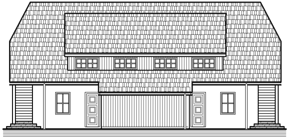
JIHOZÁPADNÍ POHLED
