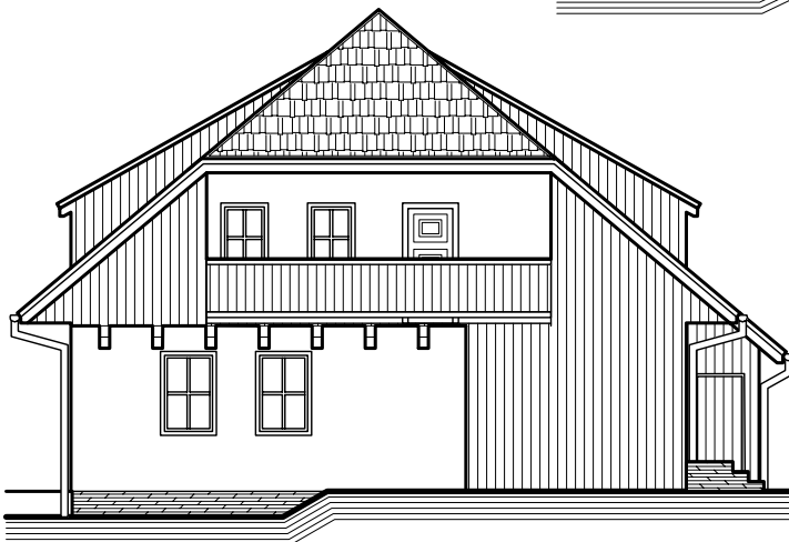
SEVEROZÁPADNÍ POHLED
