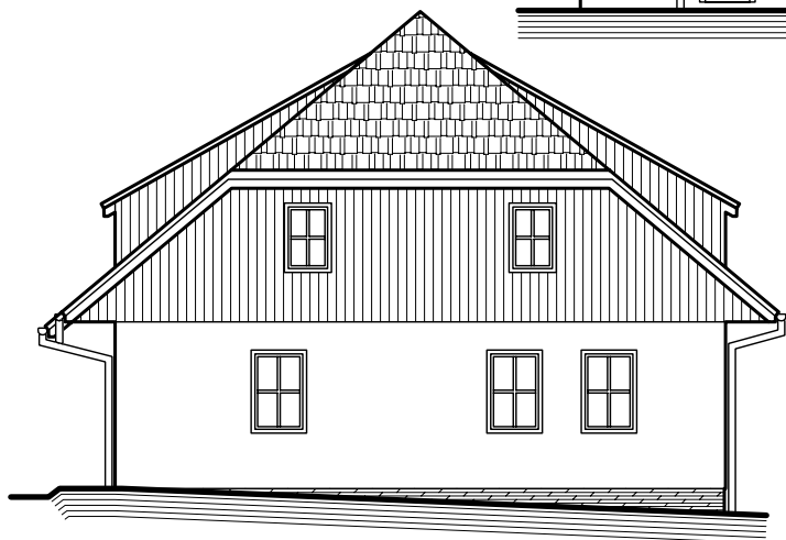
JIHOZÁPADNÍ POHLED
