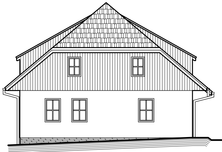
SEVEROVÝCHODNÍ POHLED
